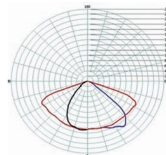
ΔΙΑΓΡΑΜΜΑ ΚΑΤΑΝΟΜΗΣ ΦΩΤΟΣ
